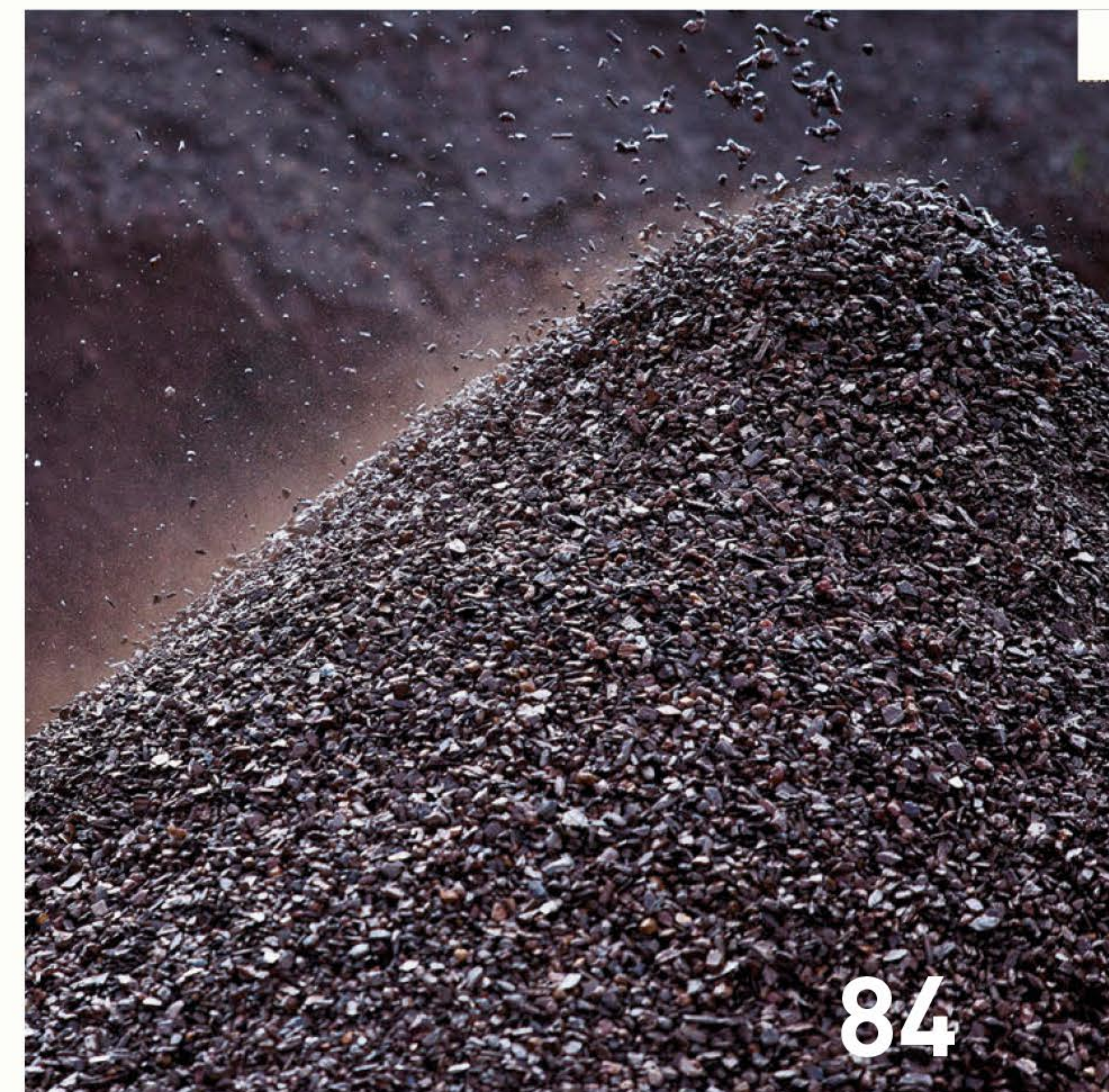
Ein Haufen Kohle: Der ungebremste Rohstoffverbrauch befeuert den Klimawandel.
